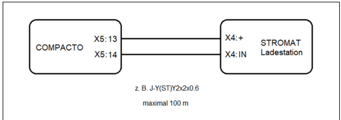
Abb. 4: Signalaustausch
