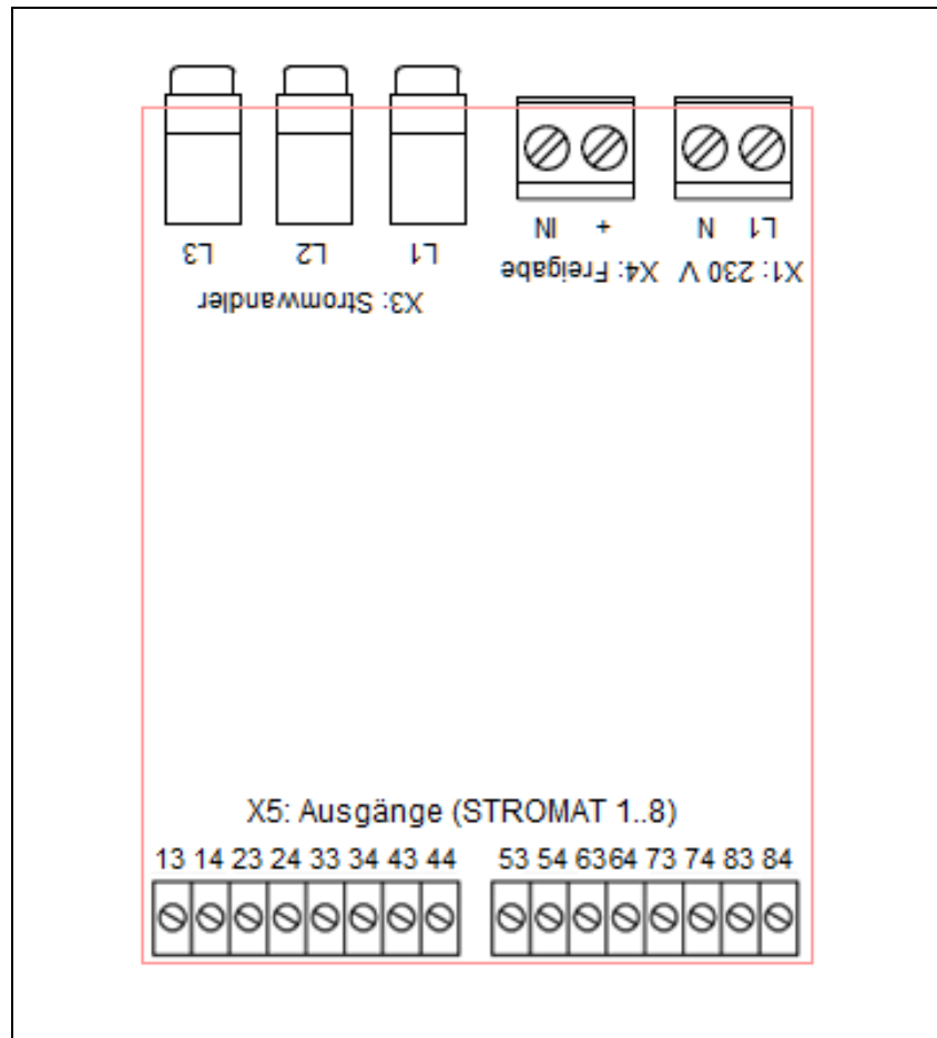
Abb. 3: COMPACTO Anschluss
