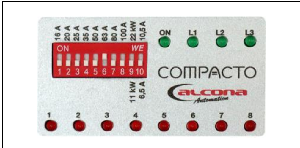
Abb. 1: COMPACTO Bedienung
