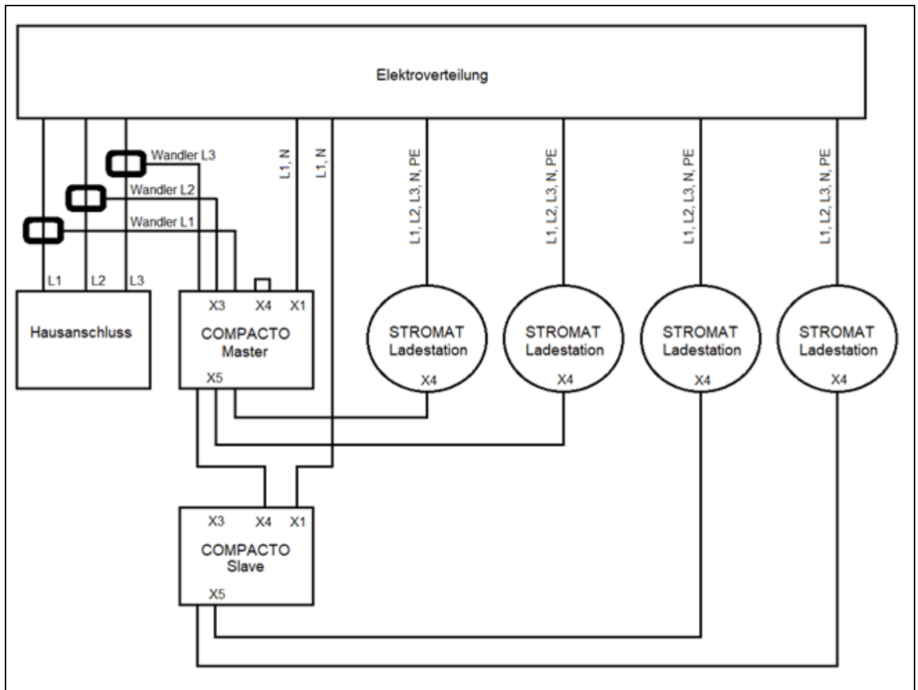
Abb. 5: Vernetzungsbeispiel
